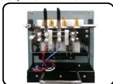
120A 単相/三相3線 下穴タイプ 注6
